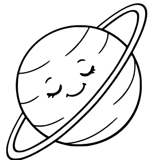
Urano
