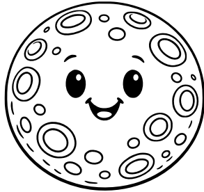
Mercurio
