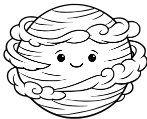
Venus
